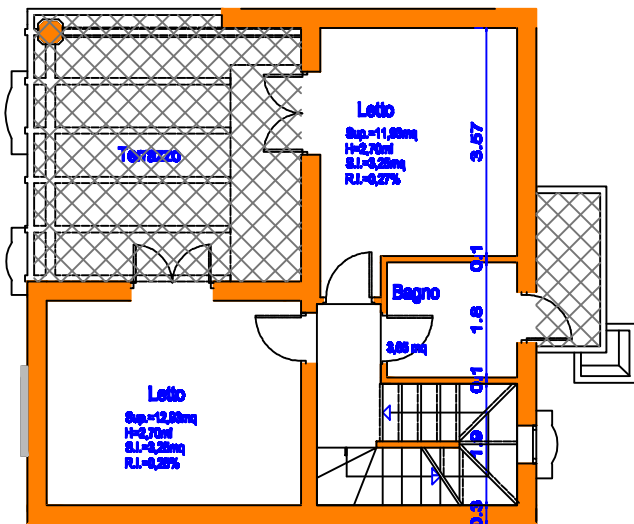
PIANO PRIMO
