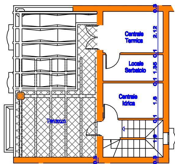
PIANO SECONDO
