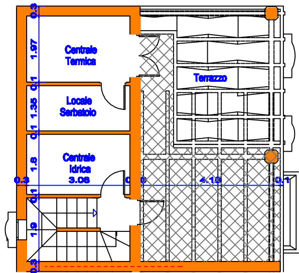
PIANO SECONDO
