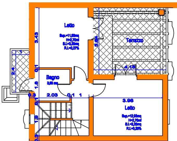
PIANO PRIMO
