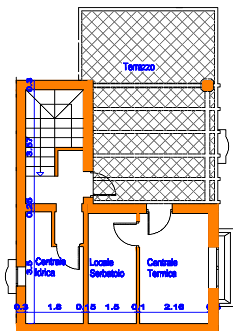
PIANO PRIMO
