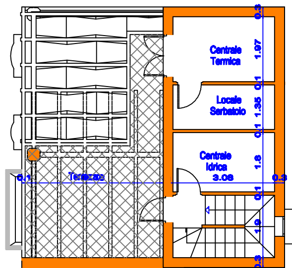
PIANO SECONDO
